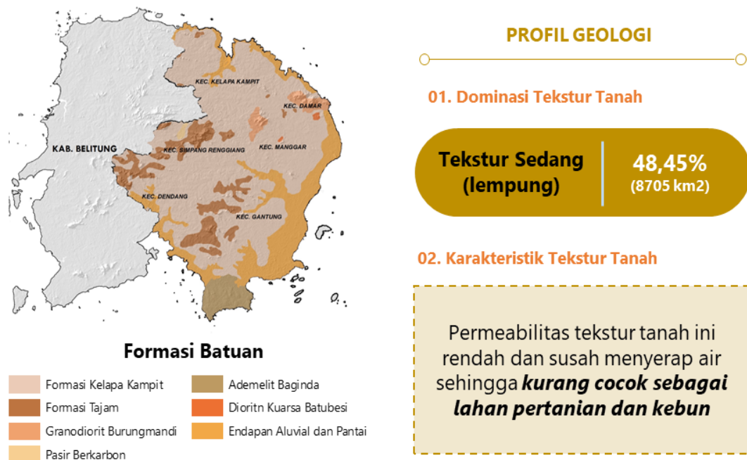
Gambar 2. 4 Kondisi Geologi Kabupaten Belitung Timur
