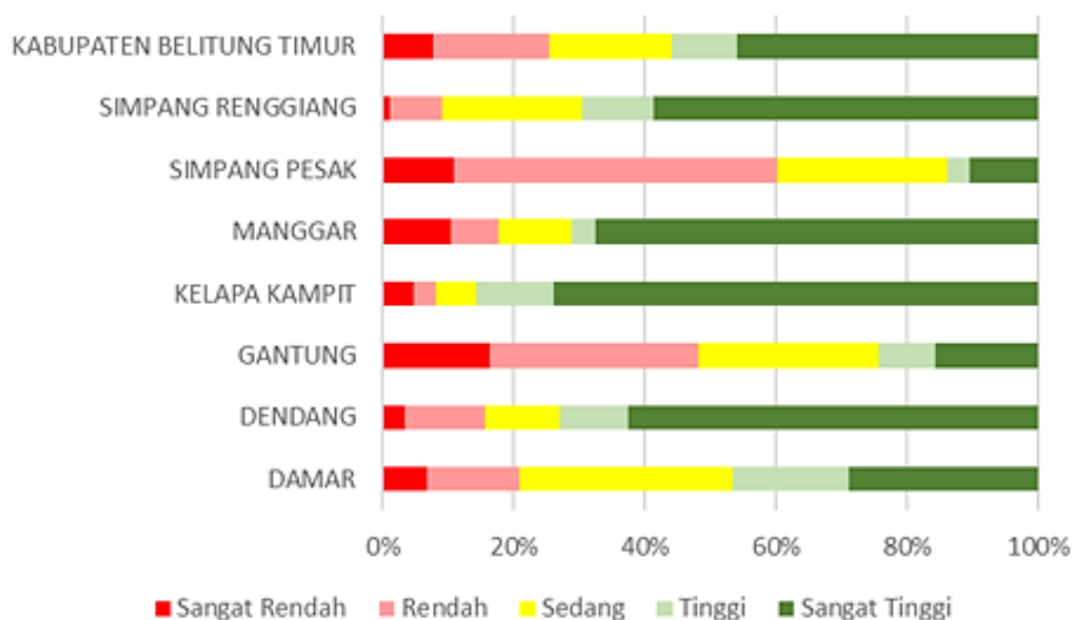
Gambar 2. 13 Persentase Kelas Jasa Ekosistem Penyedia Air Bersih
