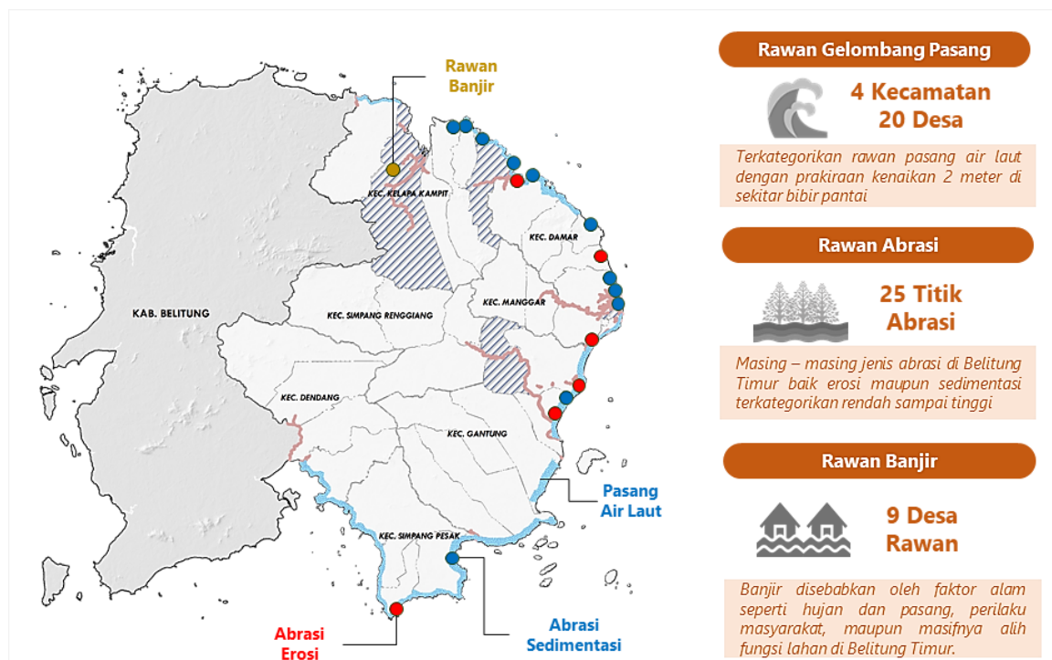
Gambar 2. 26 Kawasan Rawan Bencana Kabupaten Belitung Timur
