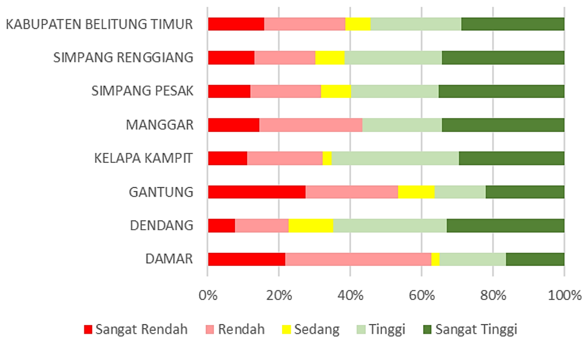
Gambar 2. 15 Persentase Kelas Jasa Ekosistem Pengolahan dan Penguraian Limbah
