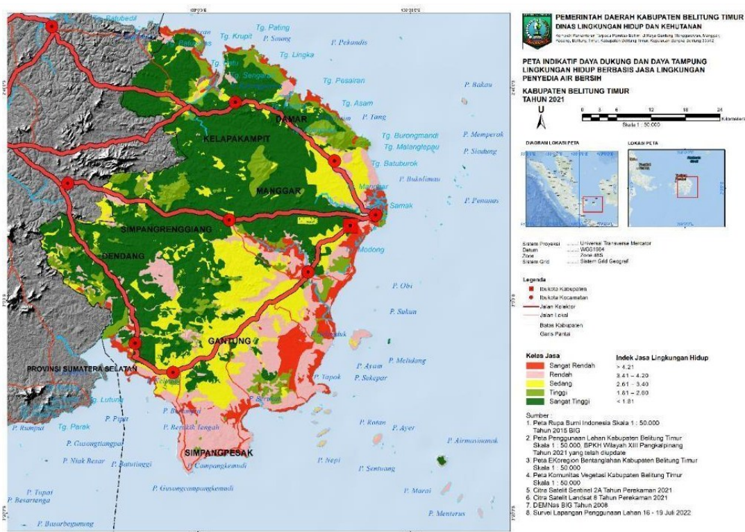
Gambar 2. 14 Peta Daya Dukung dan Daya Tampung Berbasis Jasa Ekosistem Penyedia Air Bersih
